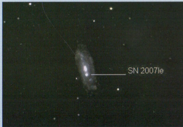
SN2007le szupernova
